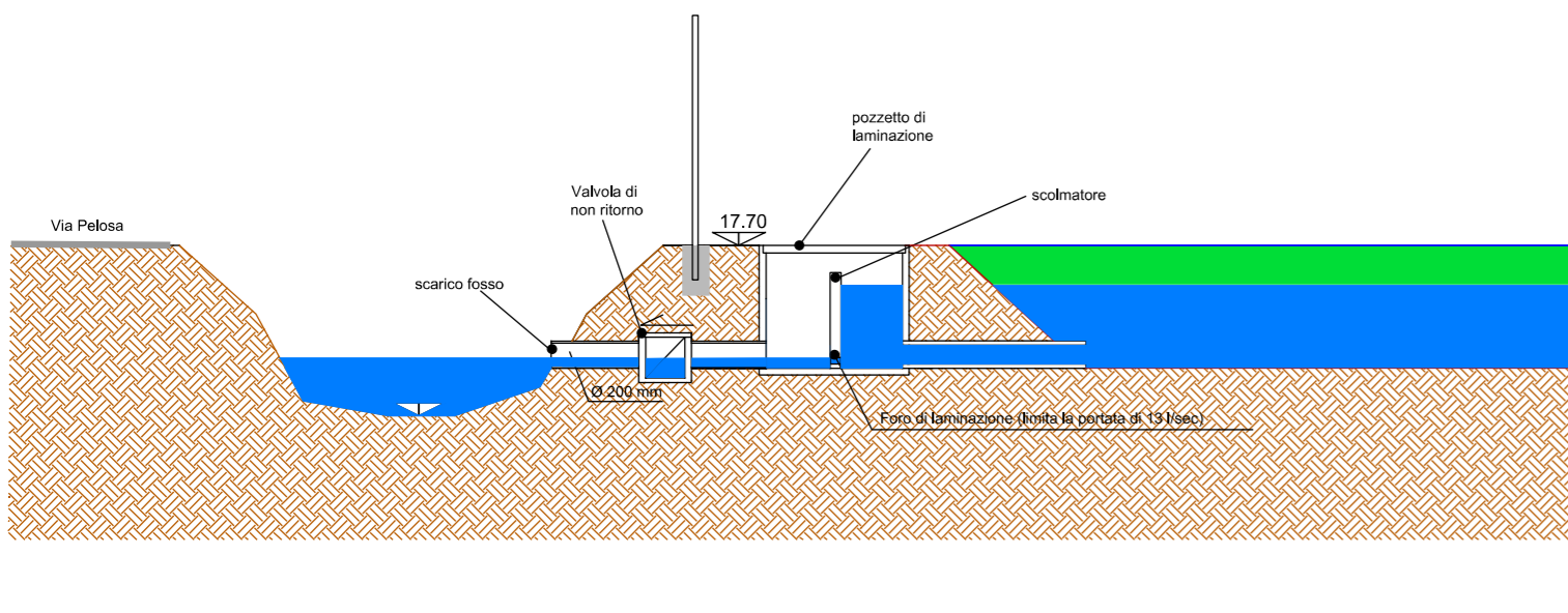
Sezione di massima manufatto di restituzione
